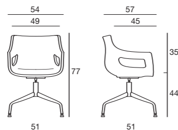
con cuscino H seduta 46 cm | seat with cushion H 46 cm
